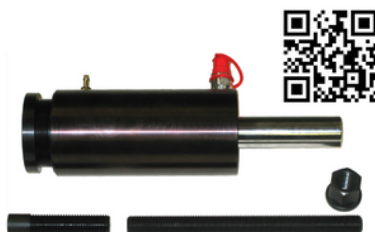
32 tonnin hydraulisylinteri pidempi vetopituus, 03-00028
